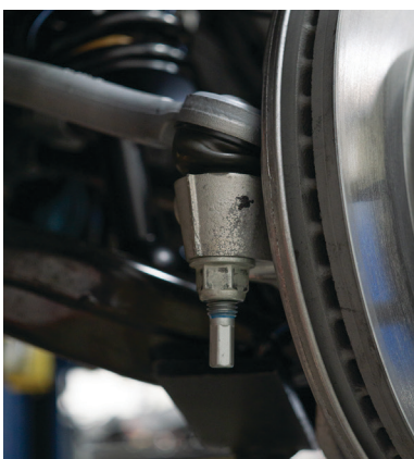
Fig. 21: Tie rod end link.
